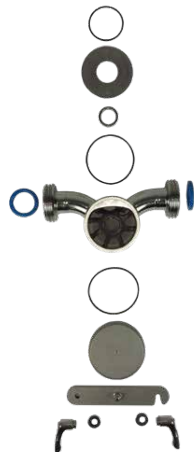
Pumpenaufbau
